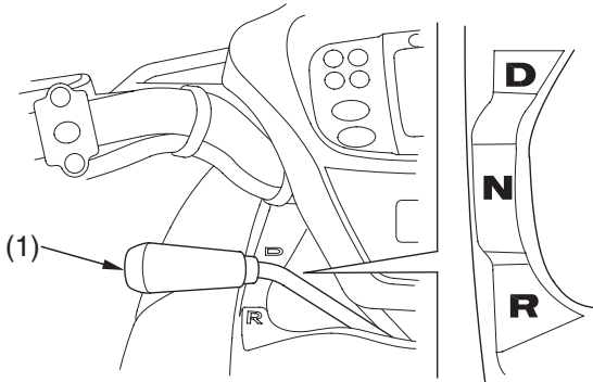
(1) shift lever
